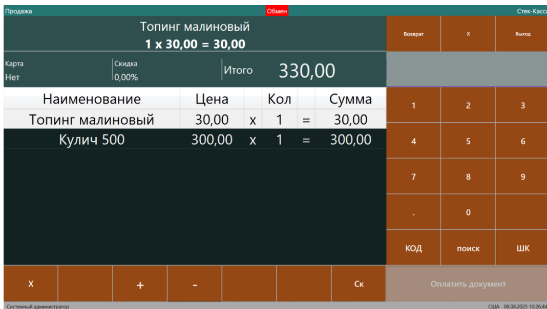
Рисунок 46 – Окно «Регистрации» с позициями
