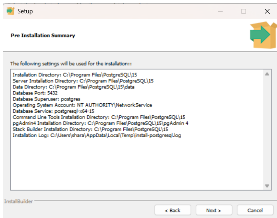
Рисунок 11 – Окно проверки данных установки
