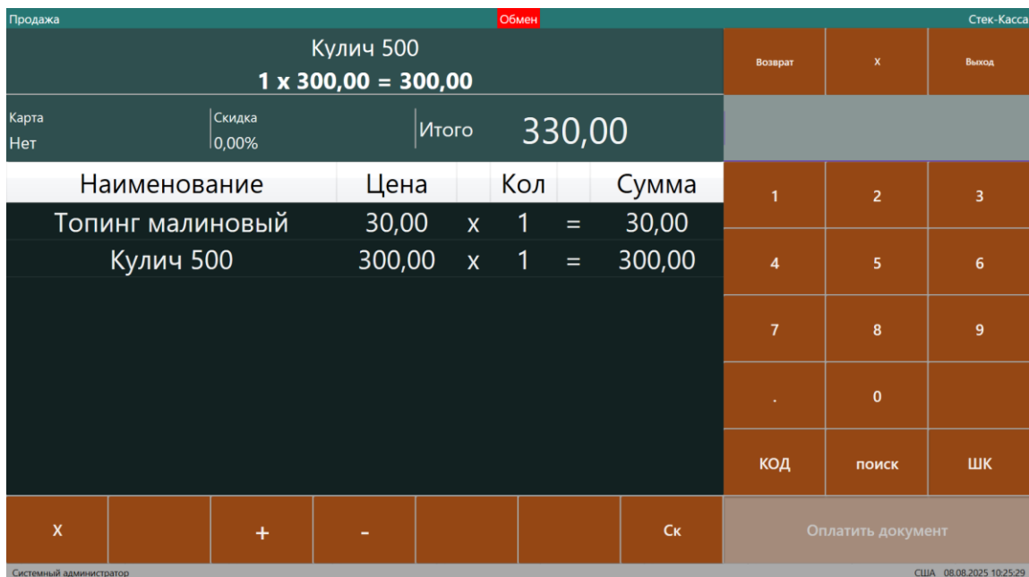
Рисунок 45 – Окно «Регистрации» с позициями
