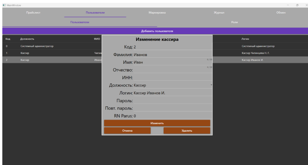
Рисунок 26 – Окно изменения пользователя
