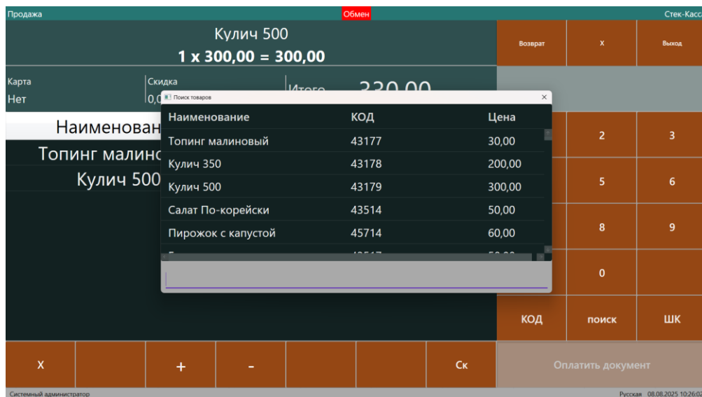
Рисунок 49 – Окно «Поиск товаров»
